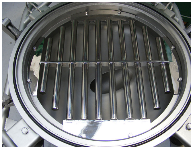
Image 2. Le séparateur magnétique, monté sur le tamiseur Blow Thru Sieve™
